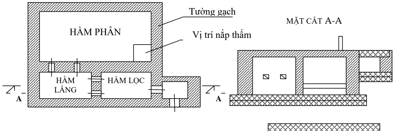
Hình 5: Cấu tạo bể tự hoại 3 ngăn
