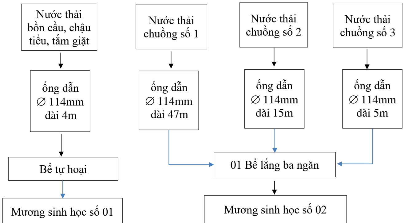
Hình 4: Sơ đồ thu gom và xử lý nước thải
