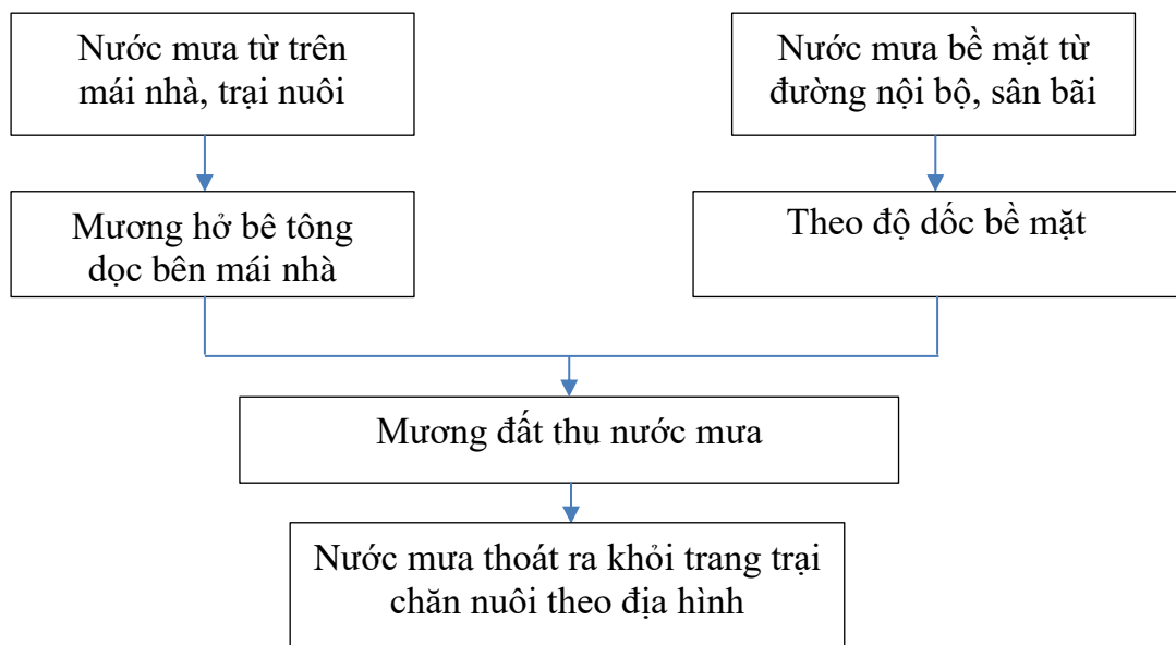
Hình 3: Sơ đồ thu gom và thoát nước mưa
