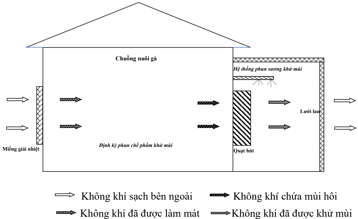
Hình 9: Hệ thống phun sương kết hợp lưới len
