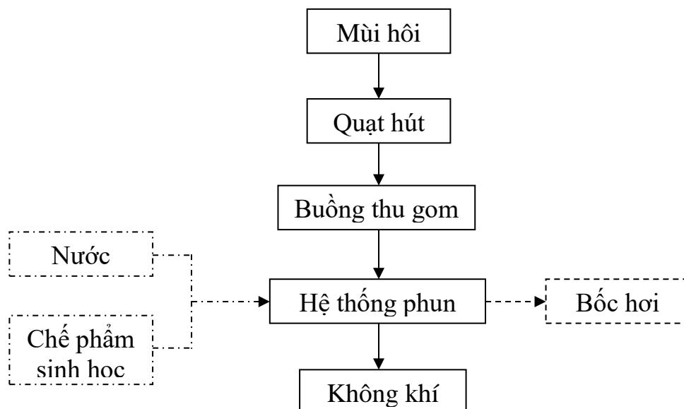
Hình 8: Sơ đồ xử lý khí thải và mùi hôi trại nuôi
