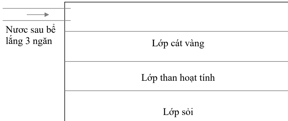
Hình 7: Cấu tạo mương sinh học
