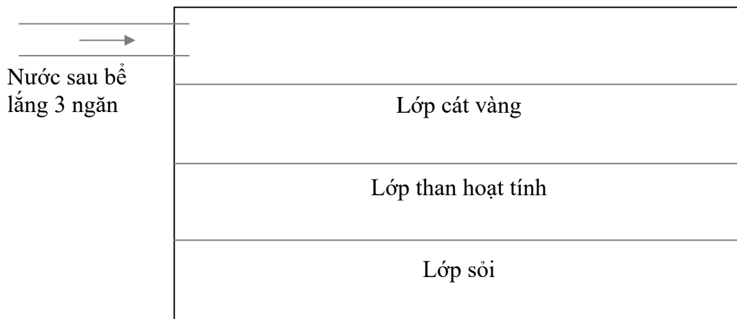
Hình 7: Cấu trúc mương sinh học
