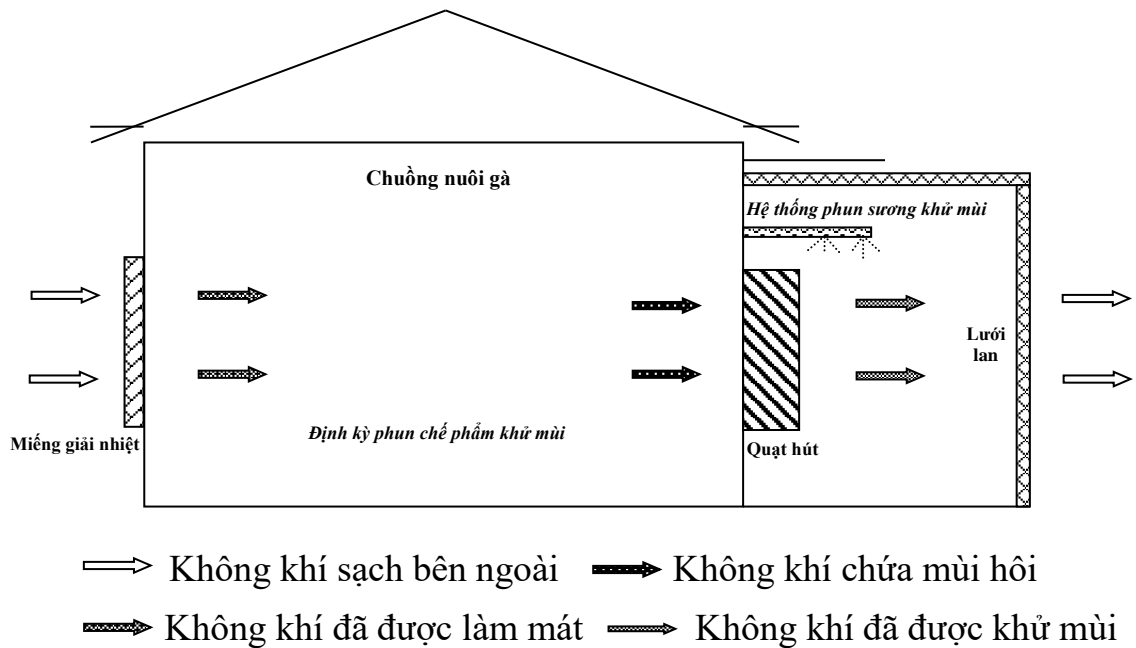
Hình 9: Hình ảnh minh họa hệ thống phun sương kết hợp lưới len
