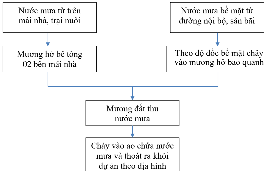
Hình 3: Sơ đồ thu gom thoát nước mưa
