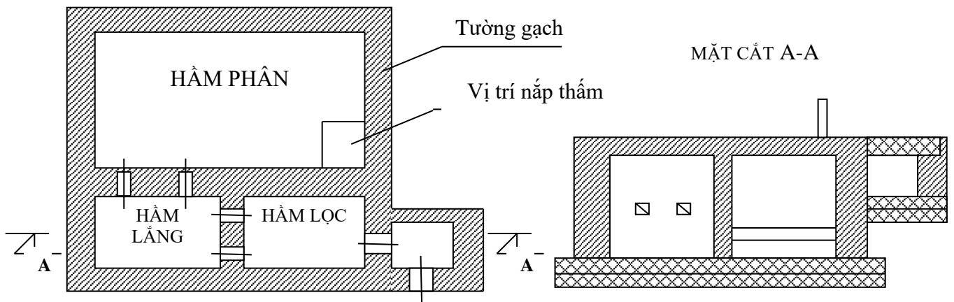
Hình 5: Cấu tạo bể tự hoại
