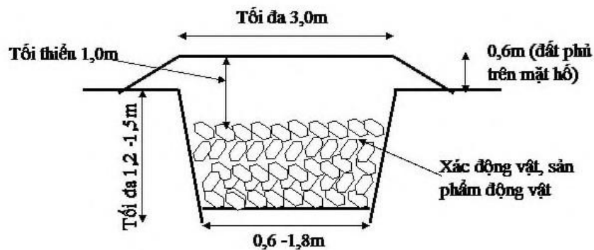
Hình 10: Mô hình hố chôn lấp gà chết do dịch bệnh
