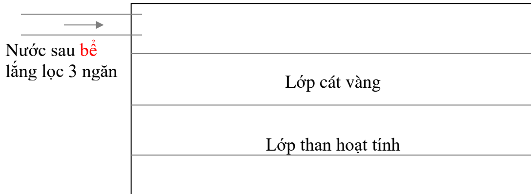
Hình 6: Sơ đồ mương sinh học
