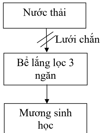
Hình 5: Quy trình hệ thống xử lý nước thải chăn nuôi
